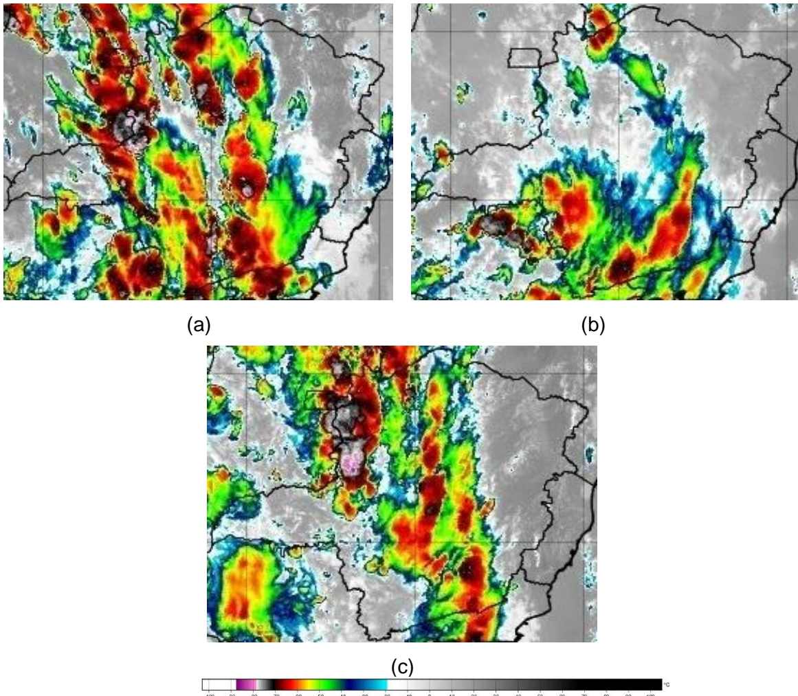
Figura 2 – Seleção de Imagem de Satélite dos dias 29 (a), 30 (b) e 31 de janeiro de 2025. Fonte: INPE.
