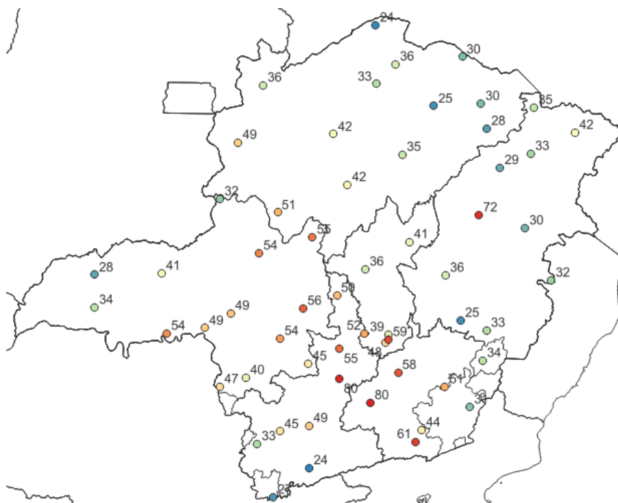
Figura 4 – Rajadas de vento (Km/h) máximas registradas entre os dias 29 e 31 de janeiro de 2025. Fonte: INMET
