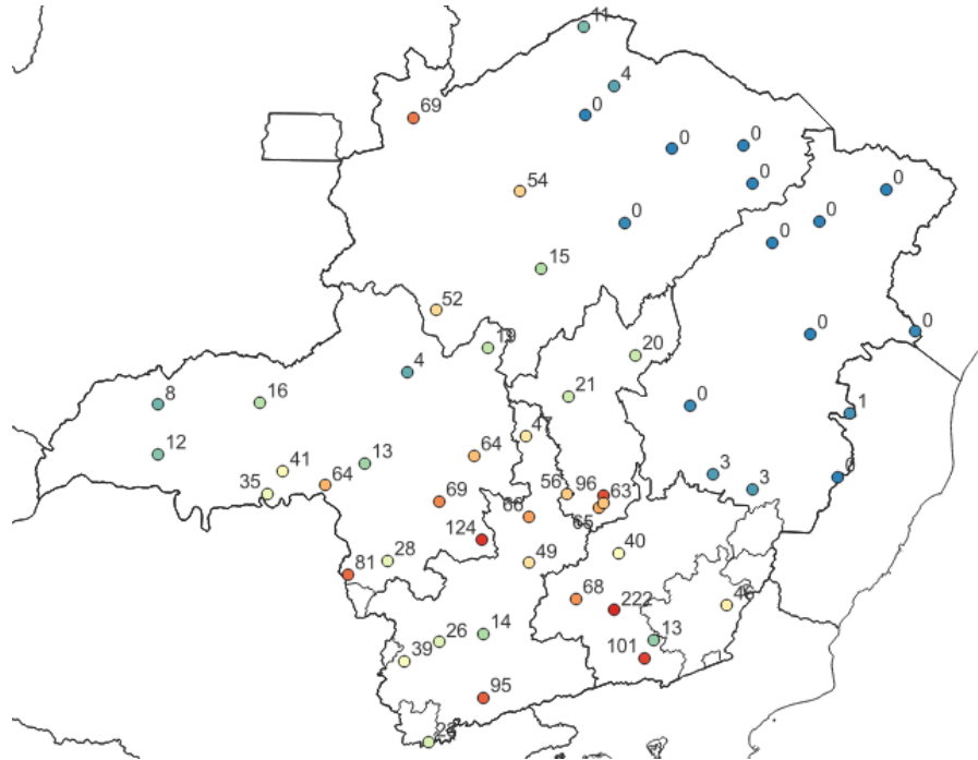
Figura 5b - Pluviometria acumulada entre os dias 29 e 31 de janeiro de 2025. Fonte dos dados: INMET.
