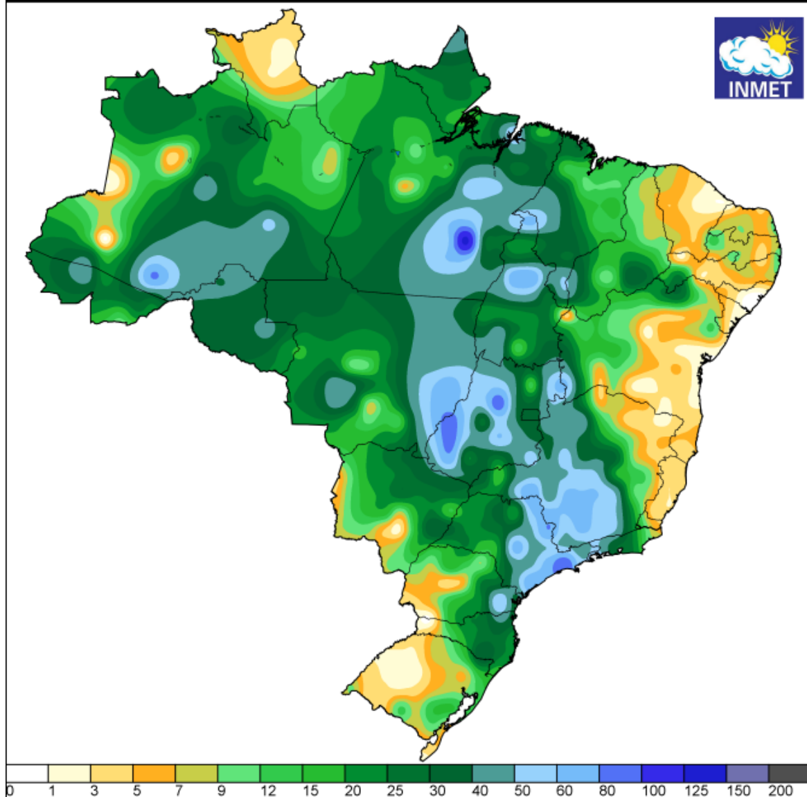
Figura 5a - Pluviometria acumulada (mm) entre os dias 29 e 31 de janeiro de 2025. Fonte: INMET.
