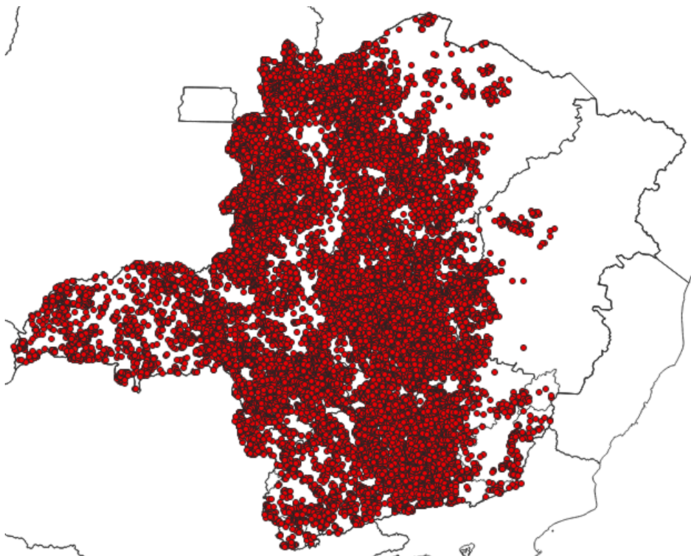
Figura 3 - Localização dos raios registrados entre os dias 29 e 31 de janeiro de 2025. Fonte: RINDAT
