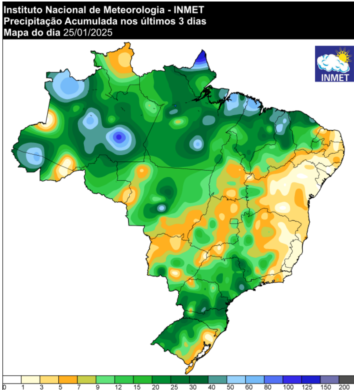
Figura 5a - Pluviometria acumulada (mm) entre os dias 22 e 24 de janeiro de 2025. Fonte: INMET.
