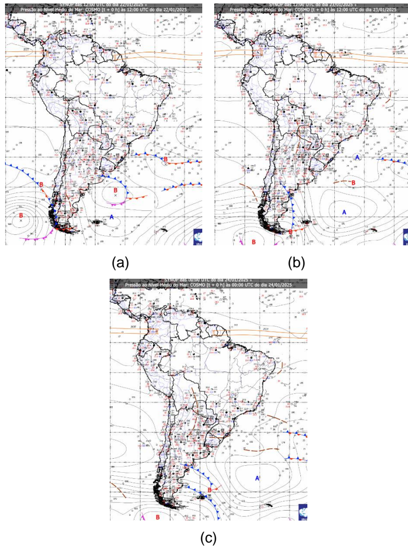
Figura 1 - Carta Sinótica em superfície dos dias 22 (a), 23 (b) e 24 (c) de janeiro de 2025. Fonte: INMET.
