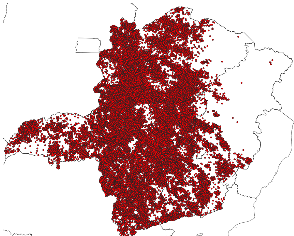
Figura 3 - Localização dos raios registrados entre os dias 22 e 24 de janeiro de 2025. Fonte: RINDAT
