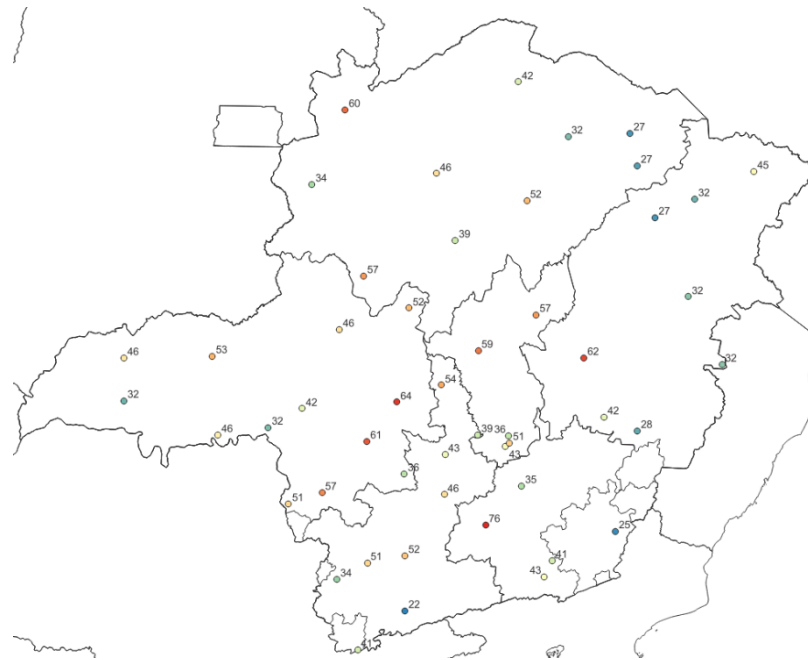
Figura 4 – Rajadas de vento (Km/h) máximas registradas entre os dias 22 e 24 de janeiro de 2025. Fonte: INMET
