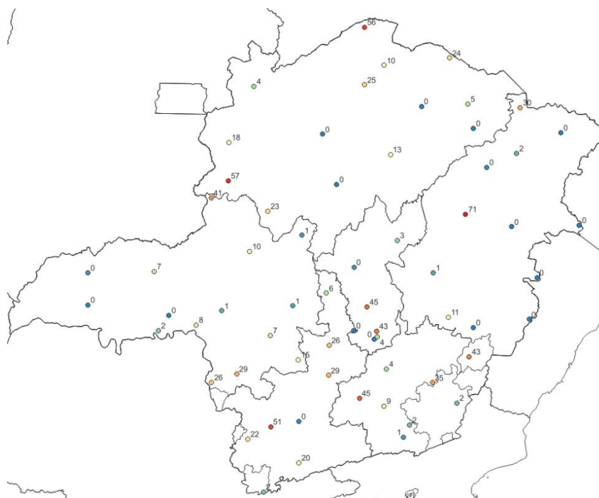
Figura 5b - Pluviometria acumulada entre os dias 22 e 24 de janeiro de 2025. Fonte dos dados: INMET.
