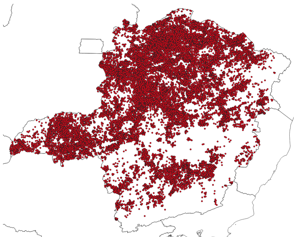
Figura 3 - Localização dos raios registrados entre os dias 21 e 23 de novembro de 2024. Fonte: RINDAT
