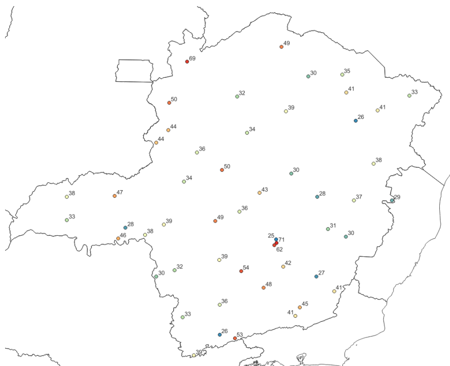
Figura 4 – Rajadas de vento (Km/h) máximas registradas entre os dias 21 e 23 de novembro de 2024. Fonte: INMET
