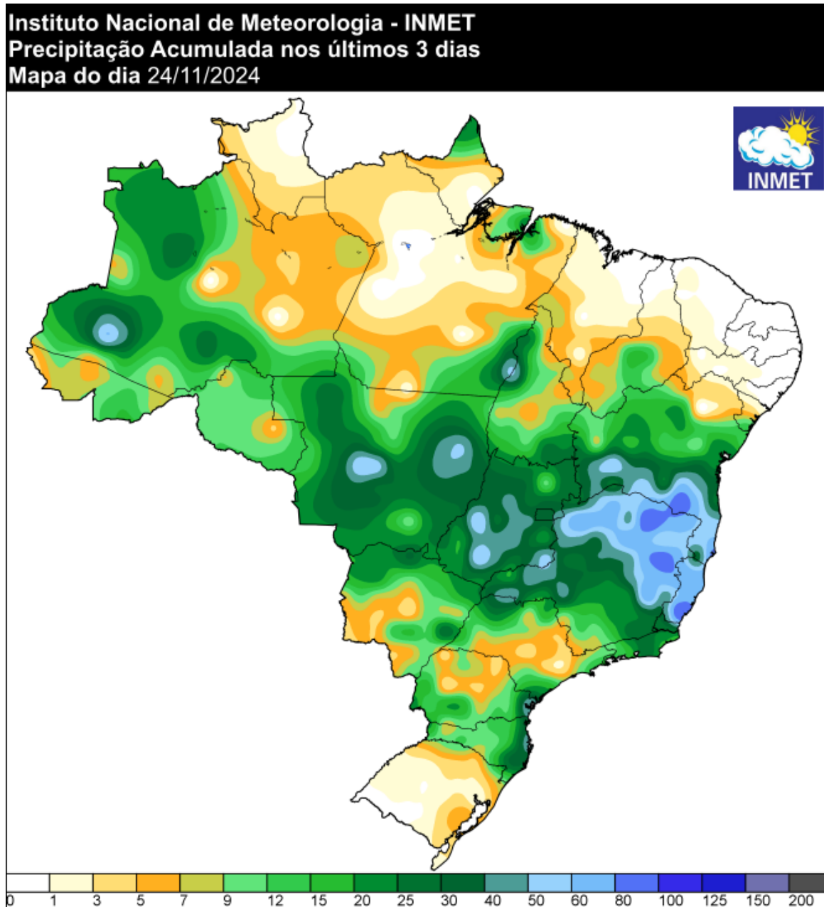
Figura 5a - Pluviometria acumulada (mm) entre os dias 21 e 23 de novembro de 2024. Fonte: INMET.
