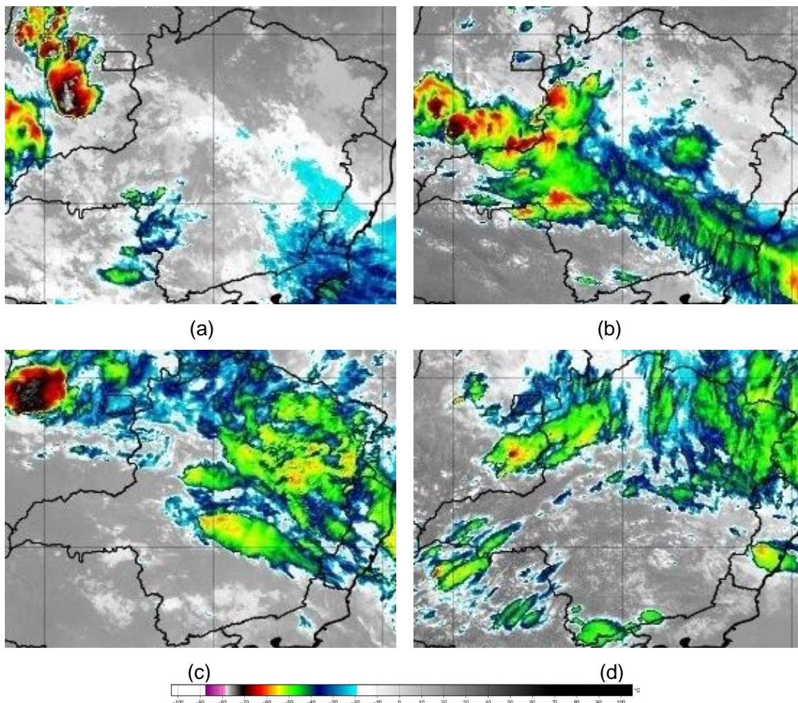
Figura 2 – Seleção de Imagens de Satélite dos dias 28 (a), 29 (b), 30 (c) e 31 (d) de outubro de 2024. Fonte: INPE.
