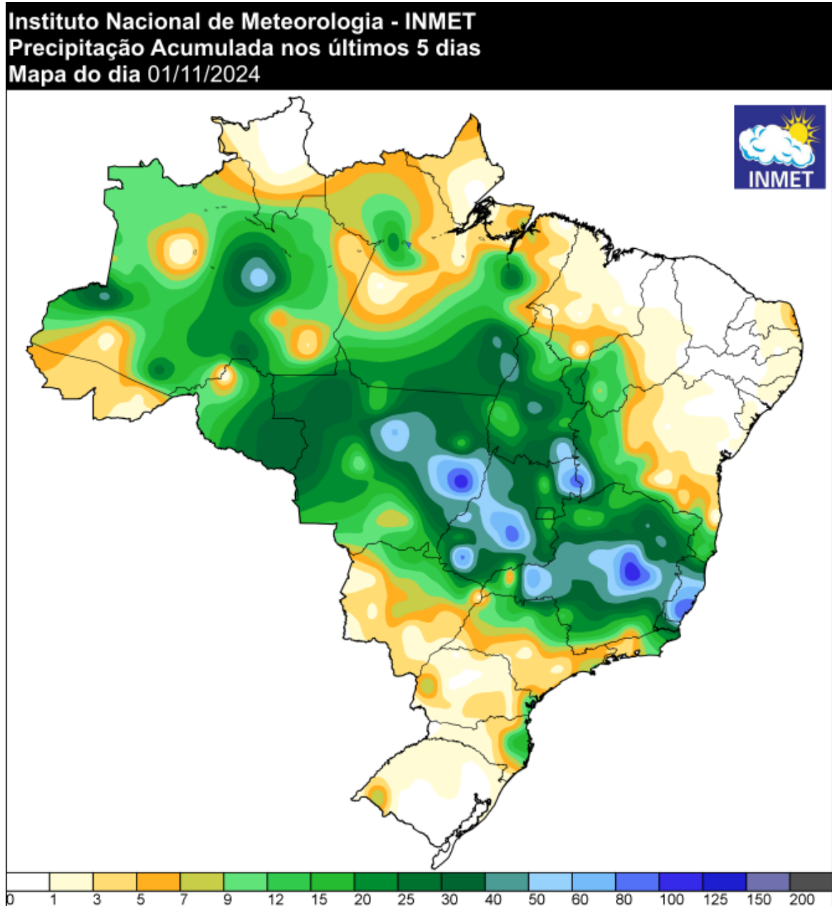
Figura 5a - Pluviometria acumulada (mm) entre os dias 27 e 31 de outubro de 2024. Fonte: INMET.
