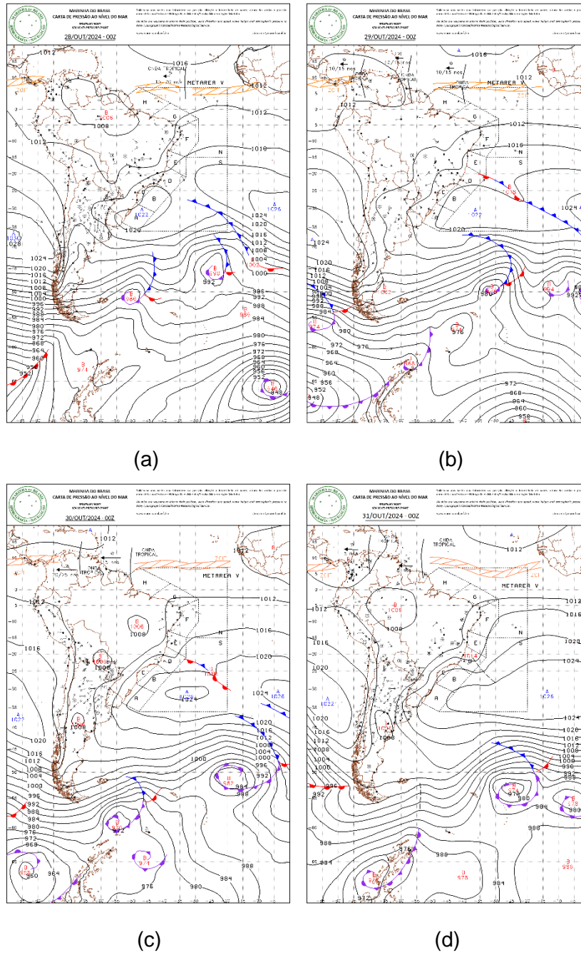
Figura 1 - Carta Sinótica em superfície dos dias 28 (a), 29 (b), 30 (c) e 31 (d) de outubro de 2024. Fonte: Marinha do Brasil.
