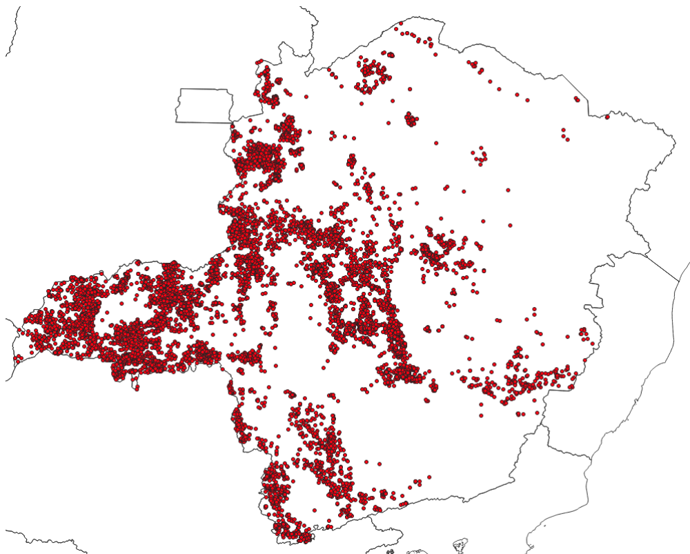
Figura 3 - Localização dos raios registrados entre os dias 28 e 31 de outubro de 2024. Fonte: RINDAT
