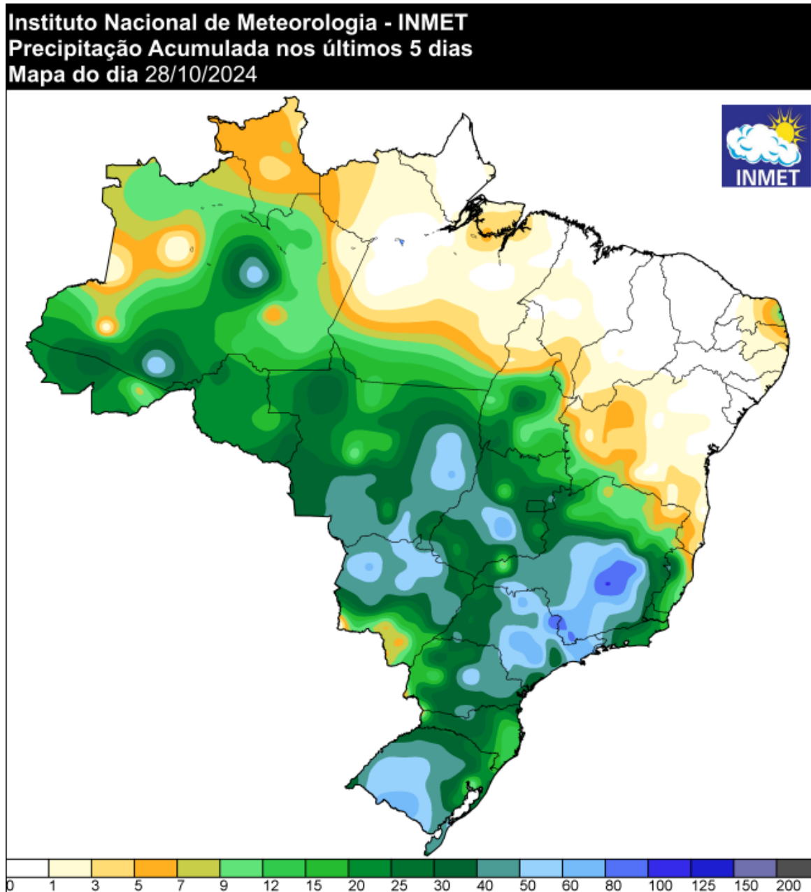
Figura 5a - Pluviometria acumulada (mm) entre os dias 23 e 27 de outubro de 2024. Fonte: INMET.
