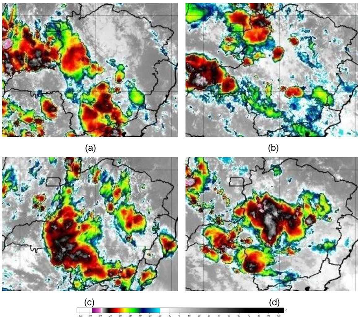
Figura 2 – Seleção de Imagens de Satélite dos dias 24 (a), 25 (b), 26 (c) e 27 (d) de outubro de 2024. Fonte: INPE.
