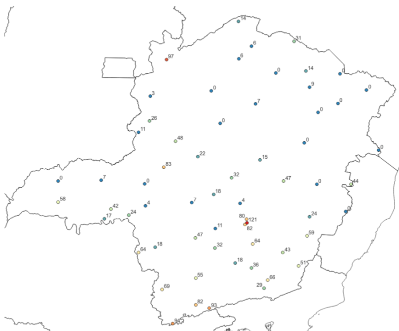
Figura 5b - Pluviometria acumulada entre os dias 24 e 27 de outubro de 2024. Fonte dos dados: INMET.
