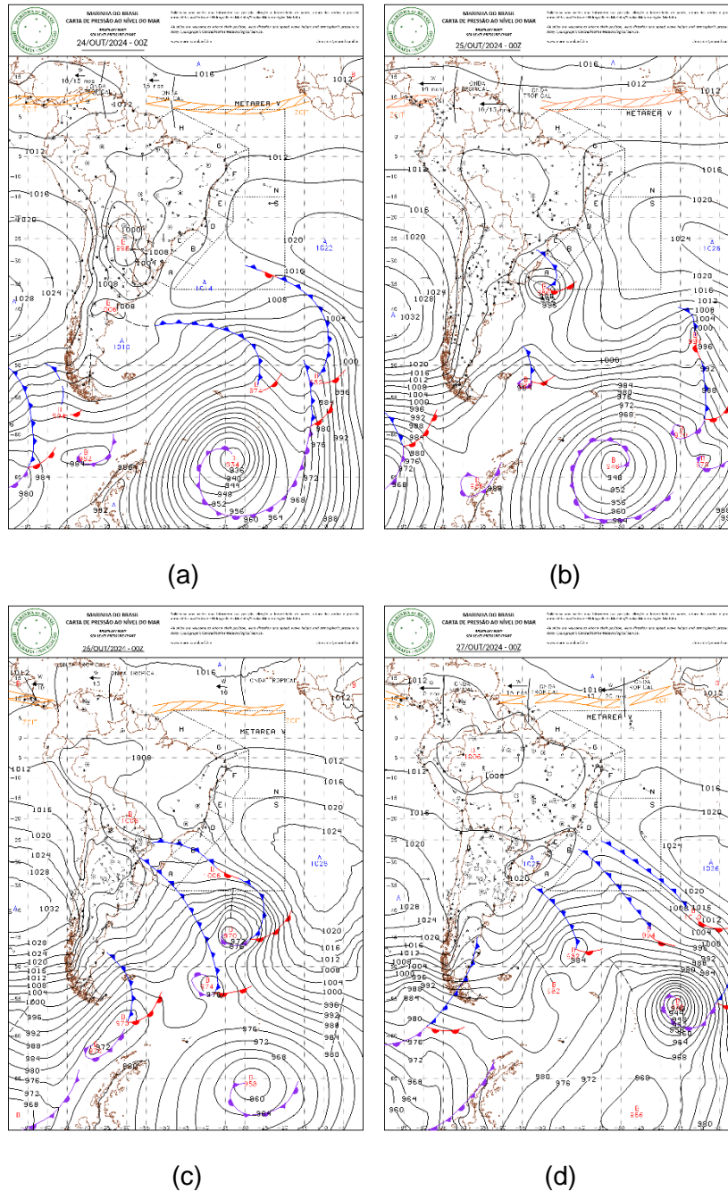
Figura 1 - Carta Sinótica em superfície dos dias 24 (a), 25 (b), 26 (c) e 27 (d) de outubro de 2024. Fonte: Marinha do Brasil.
