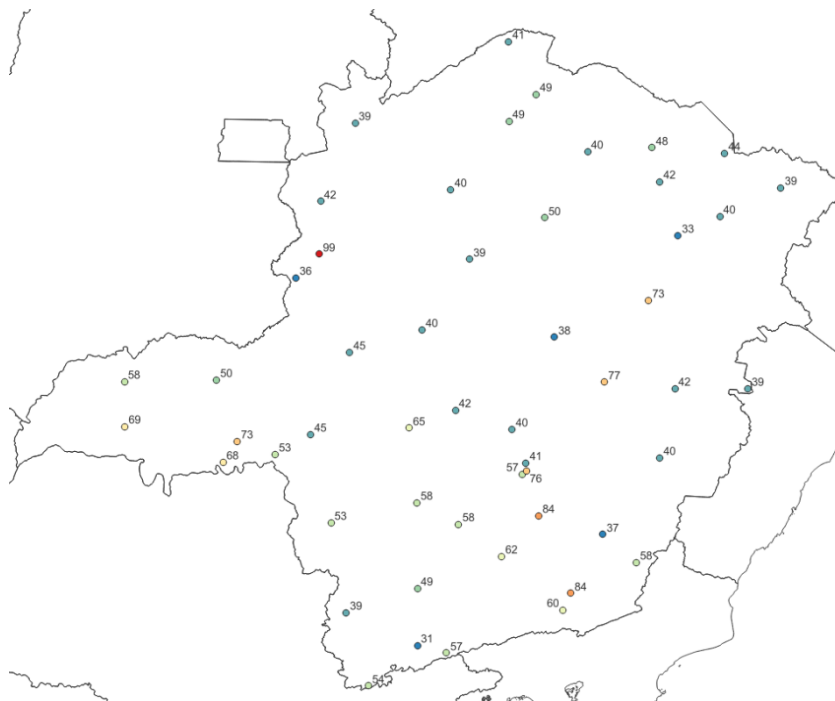
Figura 4 – Rajadas de vento (Km/h) máximas registradas entre os dias 24 e 27 de outubro de 2024. Fonte: INMET
