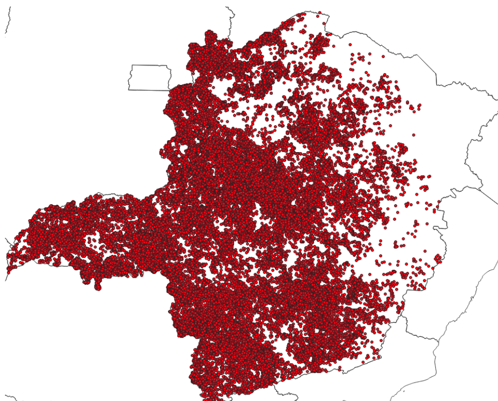
Figura 3 - Localização dos raios registrados entre os dias 24 e 27 de outubro de 2024. Fonte: RINDAT
