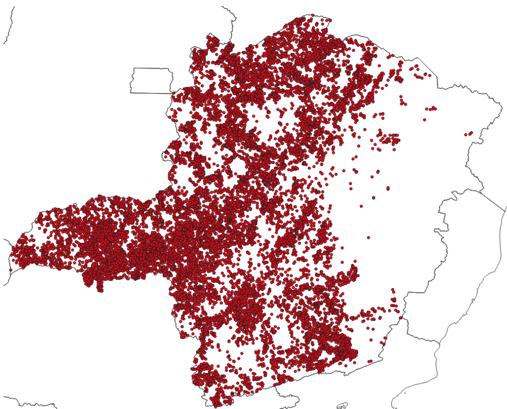
Figura 3 - Localização dos raios registrados entre os dias 17 e 21 de outubro de 2024. Fonte: RINDAT
