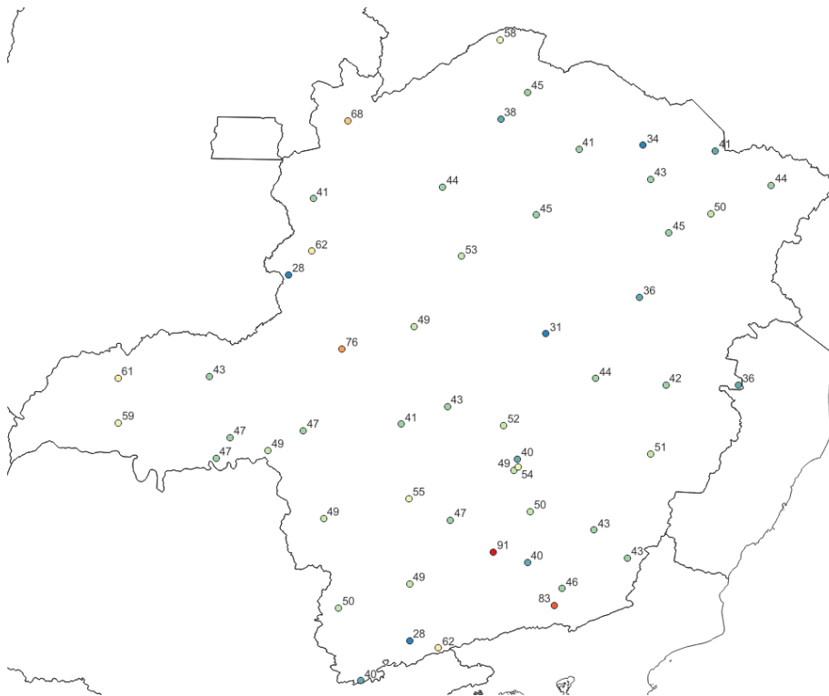
Figura 4 – Rajadas de vento (Km/h) máximas registradas entre os dias 17 e 21 de outubro de 2024. Fonte: INMET
