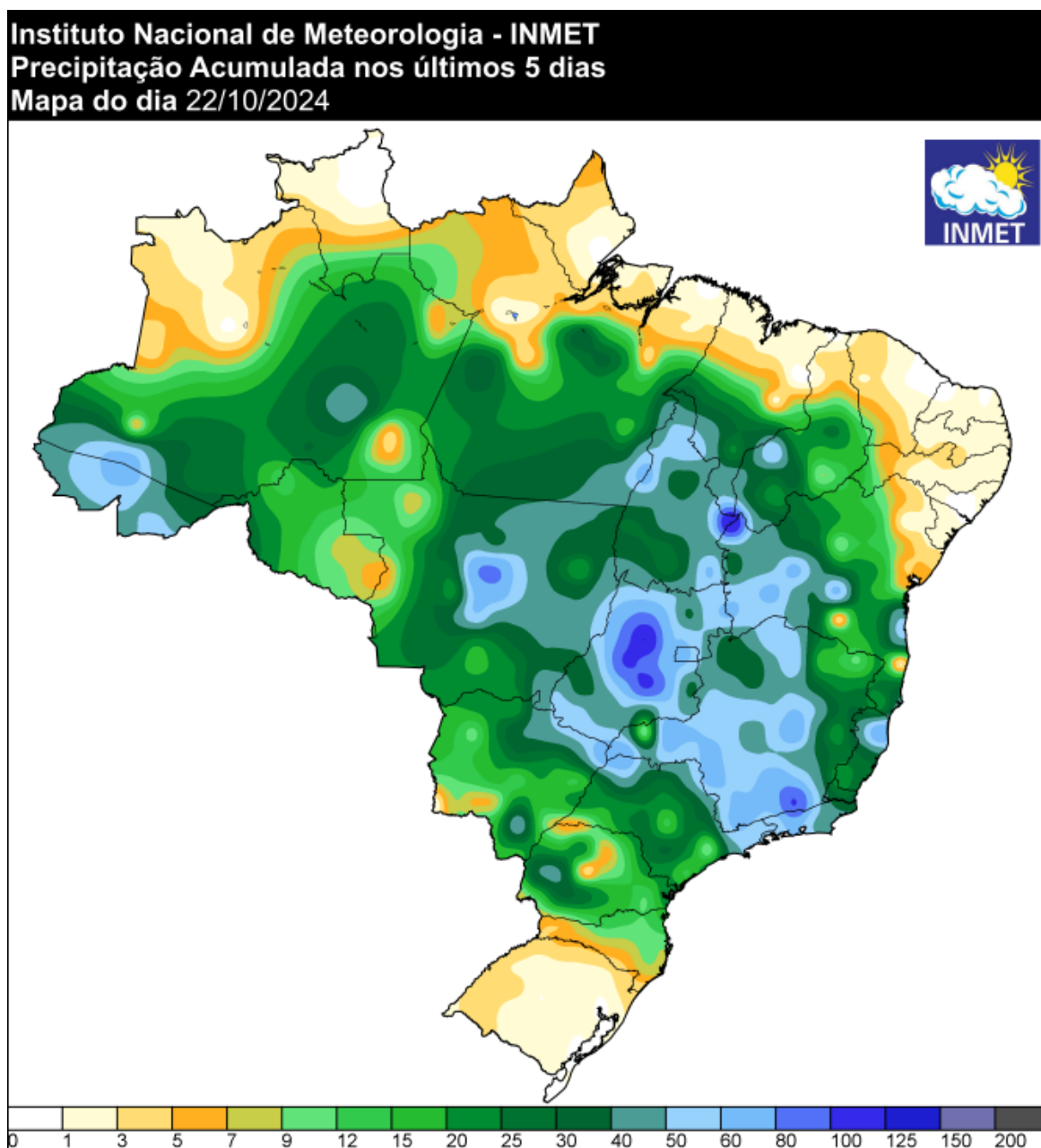
Figura 5a - Pluviometria acumulada (mm) entre os dias 17 e 21 de outubro de 2024. Fonte: INMET.
