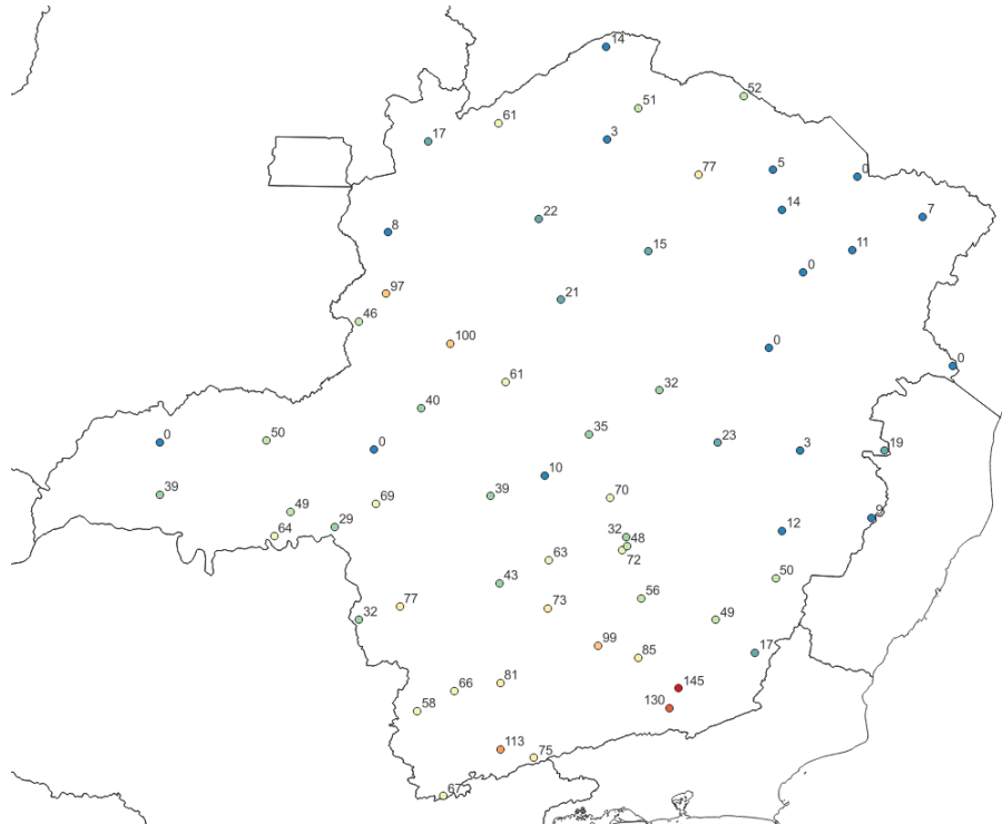
Figura 5b - Pluviometria acumulada entre os dias 17 e 21 de outubro de 2024. Fonte dos dados: INMET.
