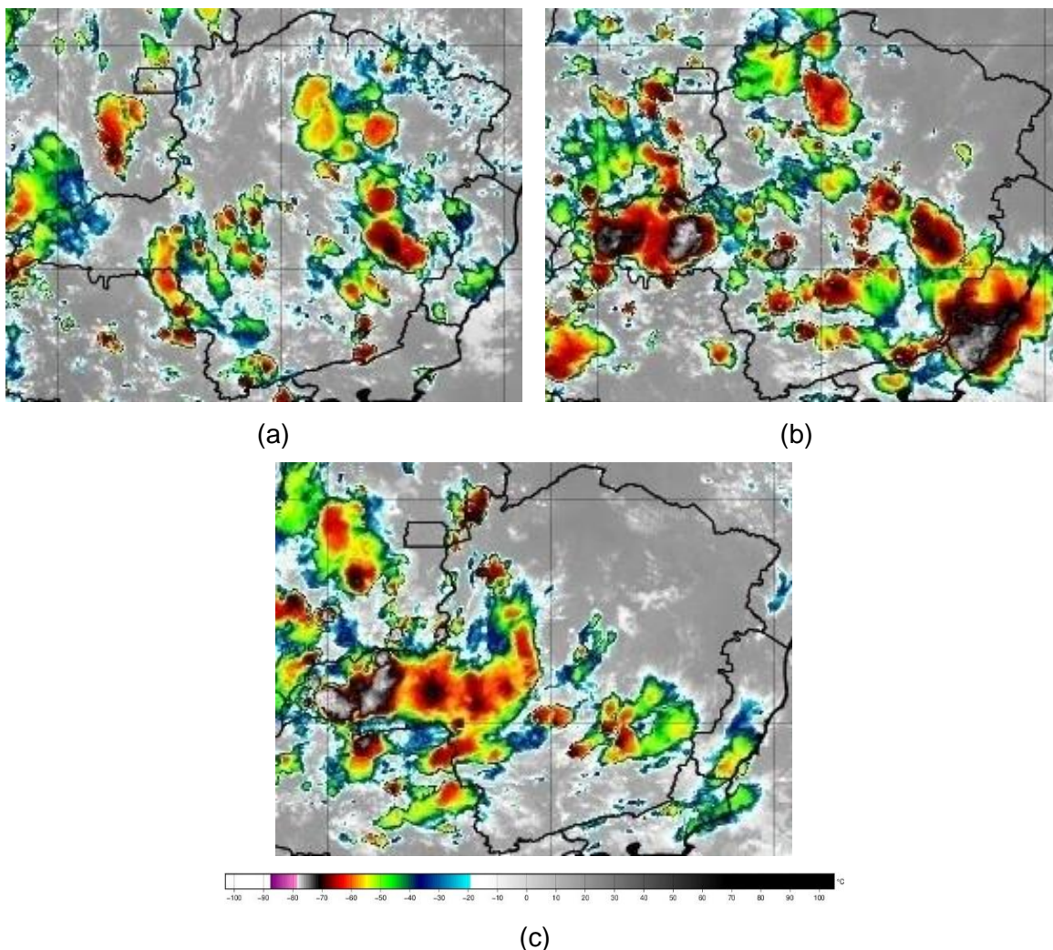
Figura 2 – Seleção de Imagem de Satélite dos dias 05 (a), 06 (b) e 07 (c) de março de 2024. Fonte: INPE.
