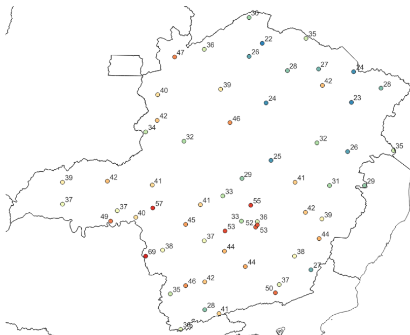
Figura 4 – Rajadas de vento (Km/h) máximas registradas entre os dias 05 e 07 de março de 2024. Fonte: INMET
