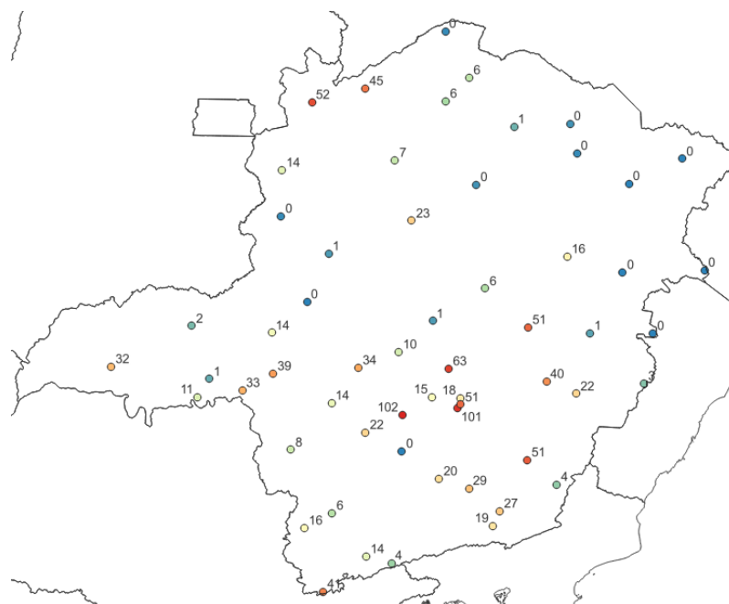
Figura 5b - Pluviometria acumulada entre os dias 05 e 07 de março de 2024. Fonte dos dados: INMET.
