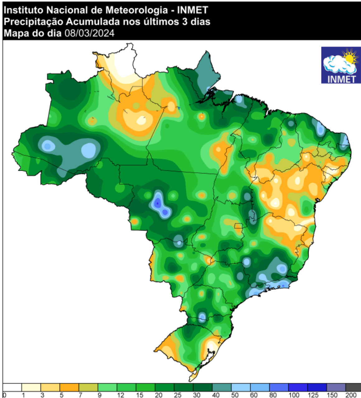
Figura 5a - Pluviometria acumulada (mm) entre os dias 05 e 07 de março de 2024. Fonte: INMET.
