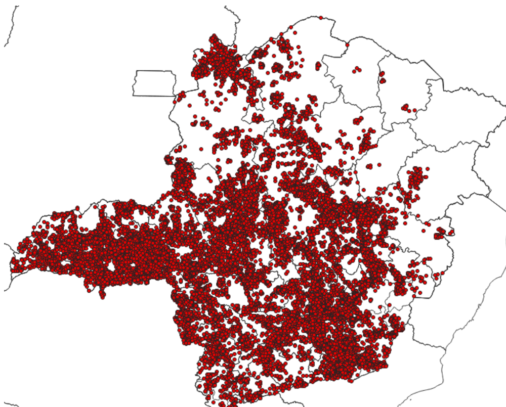
Figura 3 - Localização dos raios registrados entre os dias 05 e 07 de março de 2024. Fonte: RINDAT
