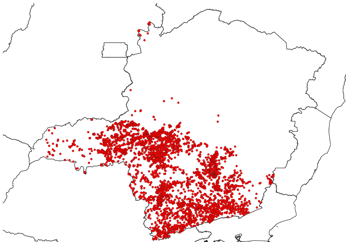
Figura 3 - Localização dos raios registrados entre os dias 25 e 27 de setembro de 2021. Fonte: RINDAT
