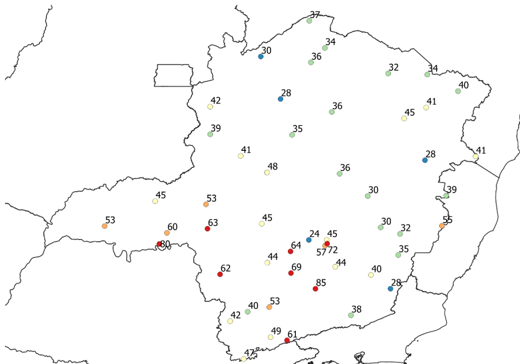
Figura 4 – Rajadas de vento máximas registradas entre os dias 25 e 27 de setembro de 2021. Fonte: INMET
