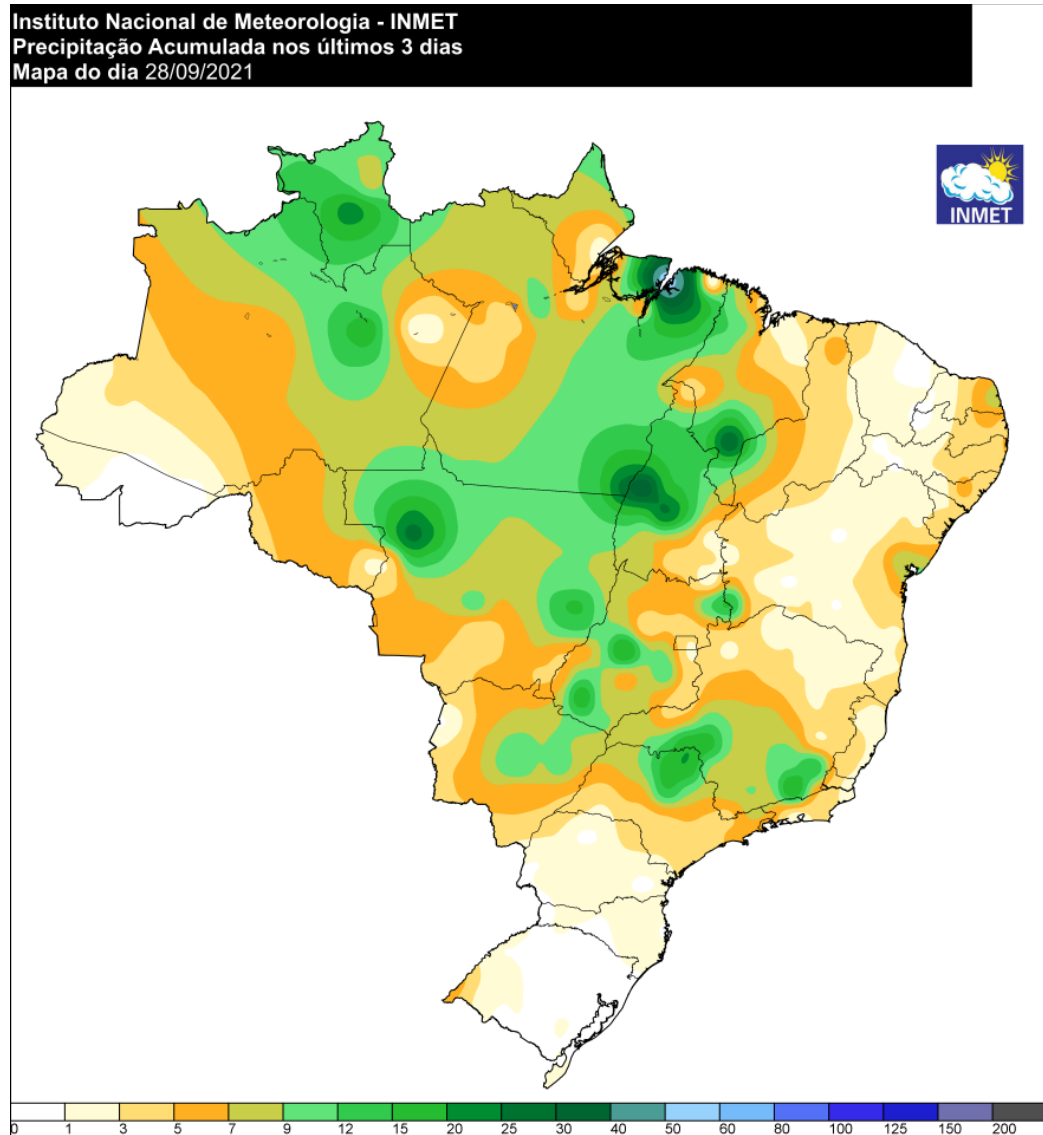
Figura 5 - Pluviometria acumulada dos dias 25 e 27 de setembro de 2021.
